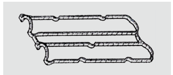
Bild 1_Zylinderkopfhaubendichtung für die Kunststoff-Zylinderkopfhaube, Reinz-Nr.: 71-38086-00, OE-Nr. 1 141 575
