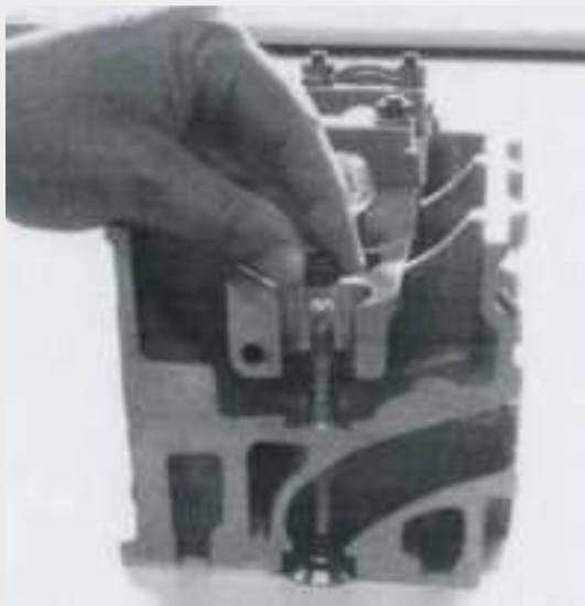
Montage mit Montagehülse
