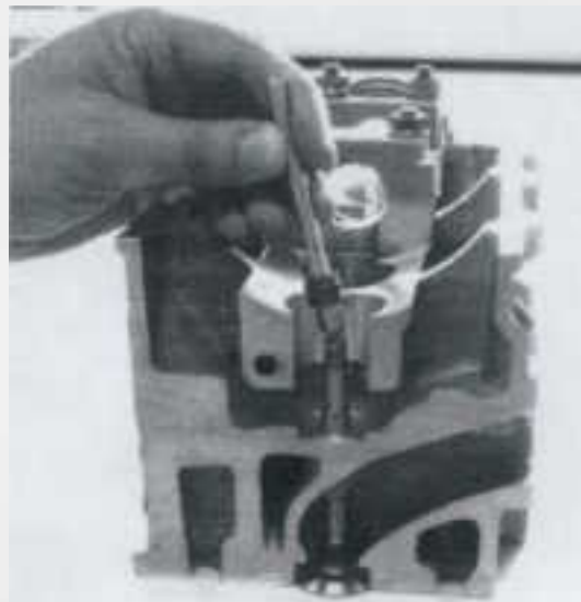
Montage mit dem Elring-Montagewerkzeug
