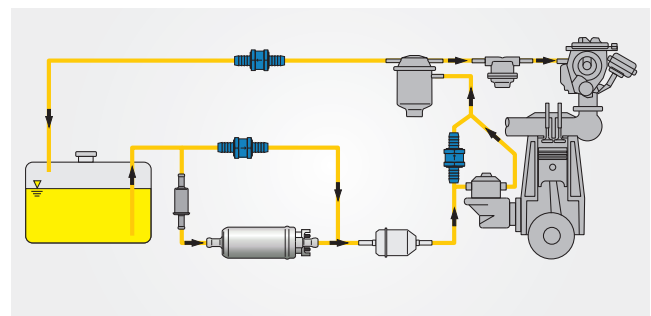
Przykład zastosowania: silnik gaźnikowy z włączaną uzupełniająco elektryczną pompą dodatkową
