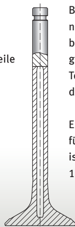
Ventilzeichnung
