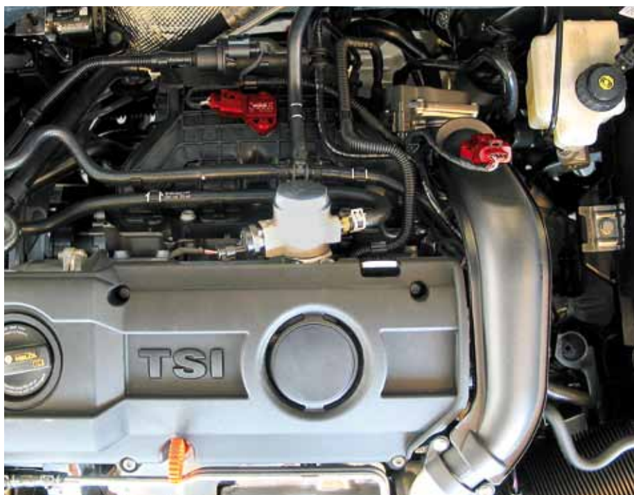
Snímač tlaku v sacím potrubí (vlevo) a snímač plnicího tlaku (vpravo) u VW Golf VI (červeně zvýrazněno)
