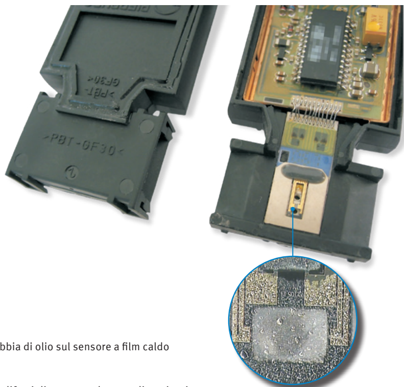
Sensore della massa dell'aria ostruito
