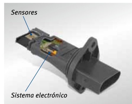
LMS de filme aquecido (versão mais recente, em corte)
