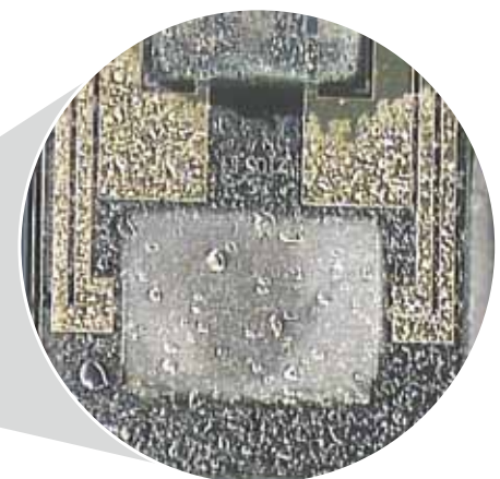
Névoa de óleo no sensor de filme aquecido
