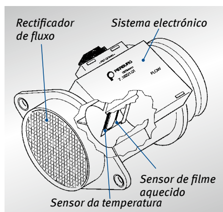
LMS de filme aquecido (versão mais antiga)
