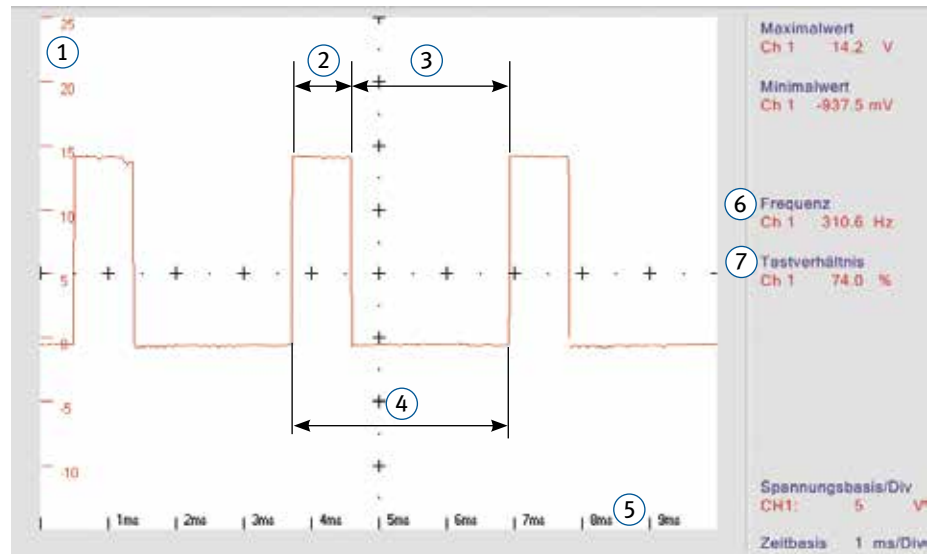
Ejemplo: Señal PWM con una relación palpadora del 74%
