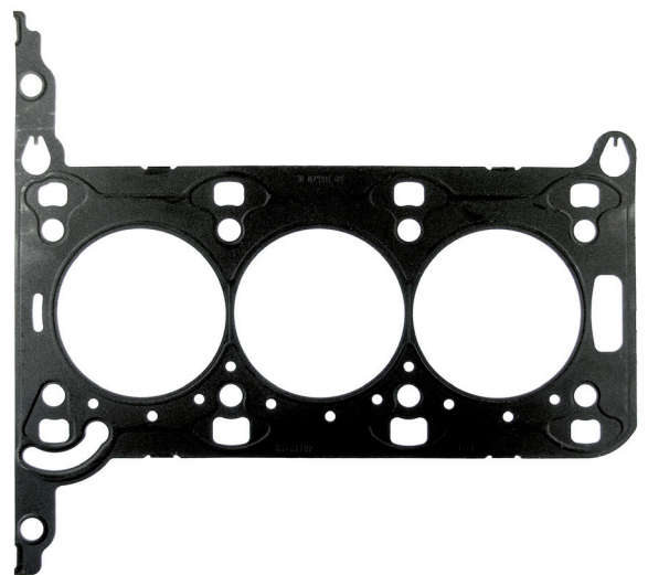
Abbildung_Zylinderkopfdichtung mit Reinz Nr. 61-37250
