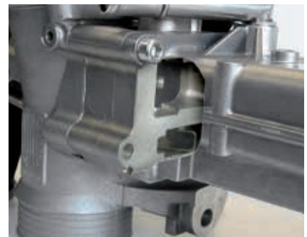
Mariposa by-pass en el radiador EGR (corte)
