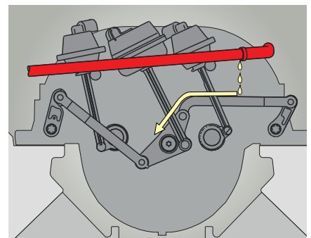
Uzrok oštećenja: Ulje curi iz voda oduška motora (istaknuto) i oštećuje polugu za prebacivanje
