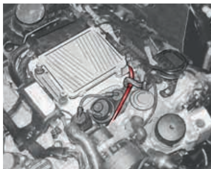
Motorni prostor W211 sa vodom oduška motora (istaknuto)
