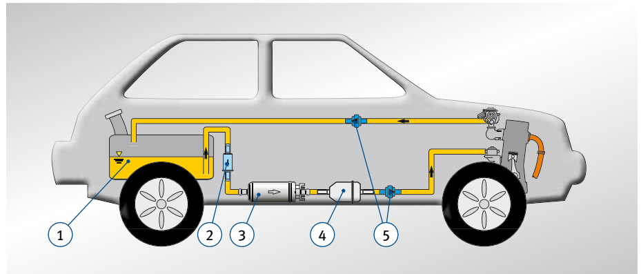
Fig. 3 : montage général
