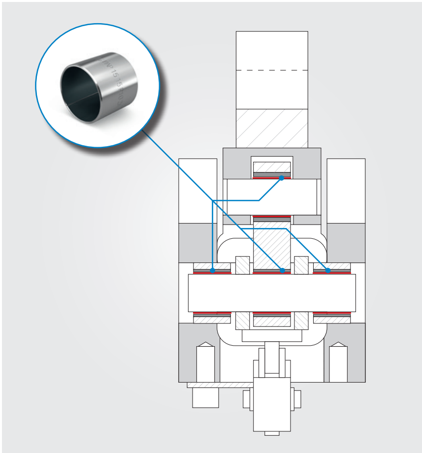
Palier d'axe dans des systèmes à genouillère avec des bagues de coussinet KS PERMAGLIDE® du type de construction PAP ... P10
