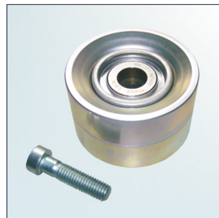
Bild 2: 532 0410 20 - neue Ausführung
