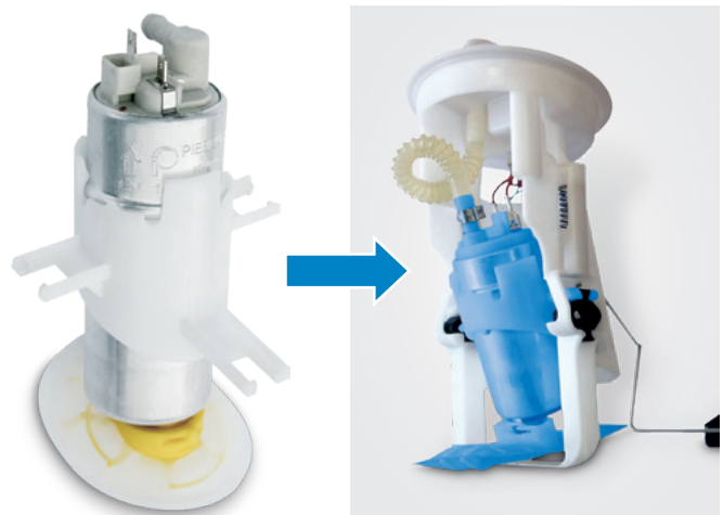
Kit de pièces de rechange pour module d'alimentation en carburant
