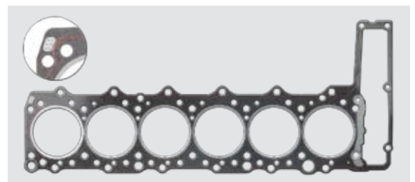
Bild 2_Neue Ausführung mit Verstärkung
