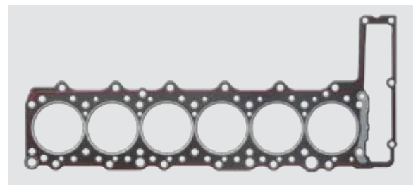
Bild 1_Alte Ausführung ohne Verstärkung
