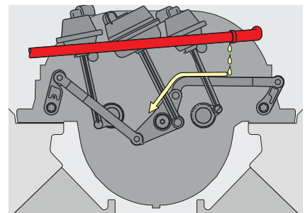
Causa de la avería: aceite sale de la tubería de la purga de aire del motor (realzada) y daña el varillaje de mando
