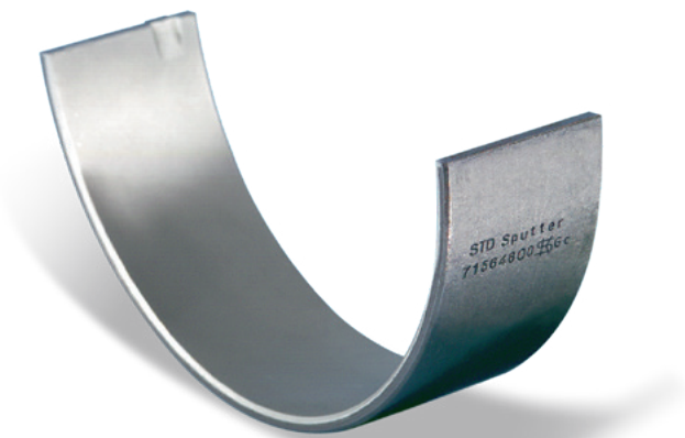
Panewka łożyska metalizowana metodą napyłania katodowego
