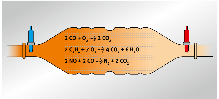
Im geregelten 3-Wege-Katalysator werden Schadstoffe durch drei chemische Reaktionen unschädlich gemacht.
