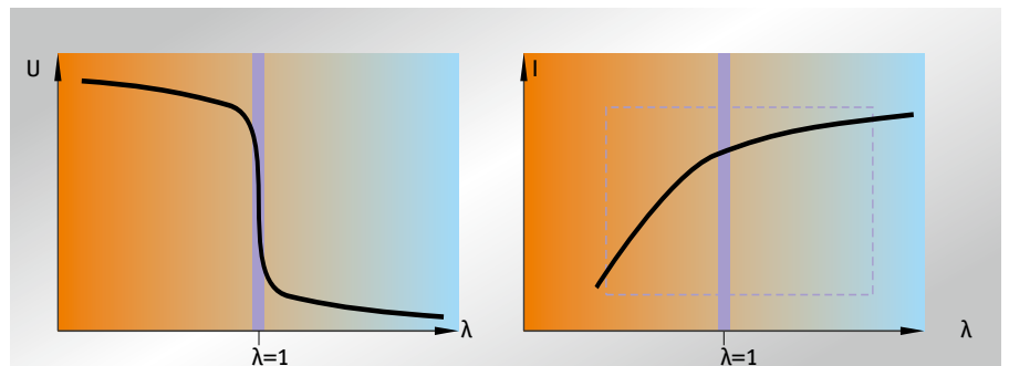
Bei „Sprungsonden“ ändert sich die Spannung um \lambda = 1 sprunghaft.
