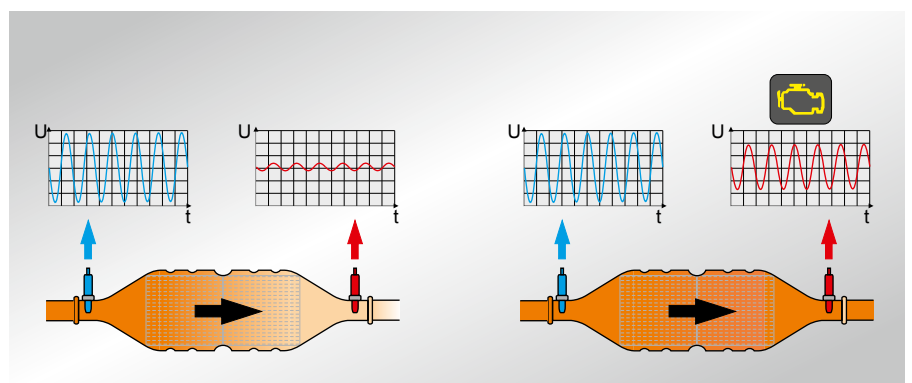
Lambdasonde als „Monitorsonde“
