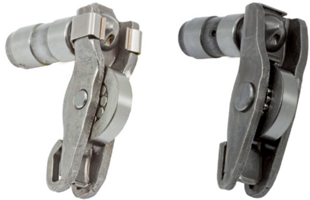
Bild 1: 423 0076 10 – Links die alte Ausführung, rechts die neue Ausführung
