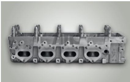
Culasse 4M41 Mitsubishi – réf. origine : 1005B341 / 1005B340
