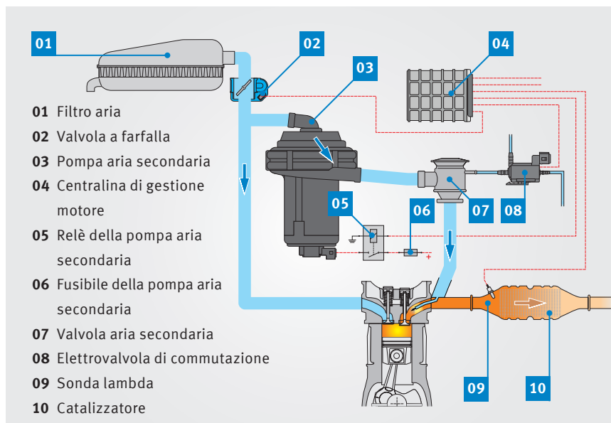
Principio dell'iniezione aria secondaria (ad azionamento pneumatico)
