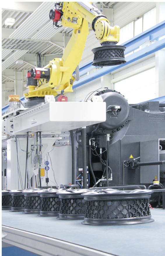
Konzeptstudie einer Pkw-Felge aus Kunststoff, gefertigt bei Hummel-Formen GmbH
