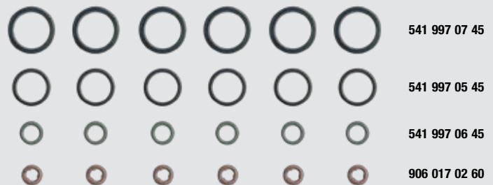
Bild2_OM 906 / OM 926, EinspritzdüSENSATZ 15-31357-03
