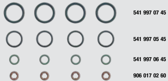
Bild1_OM 904 / OM 924, EinspritzdüSENSATZ 15-31357-02
