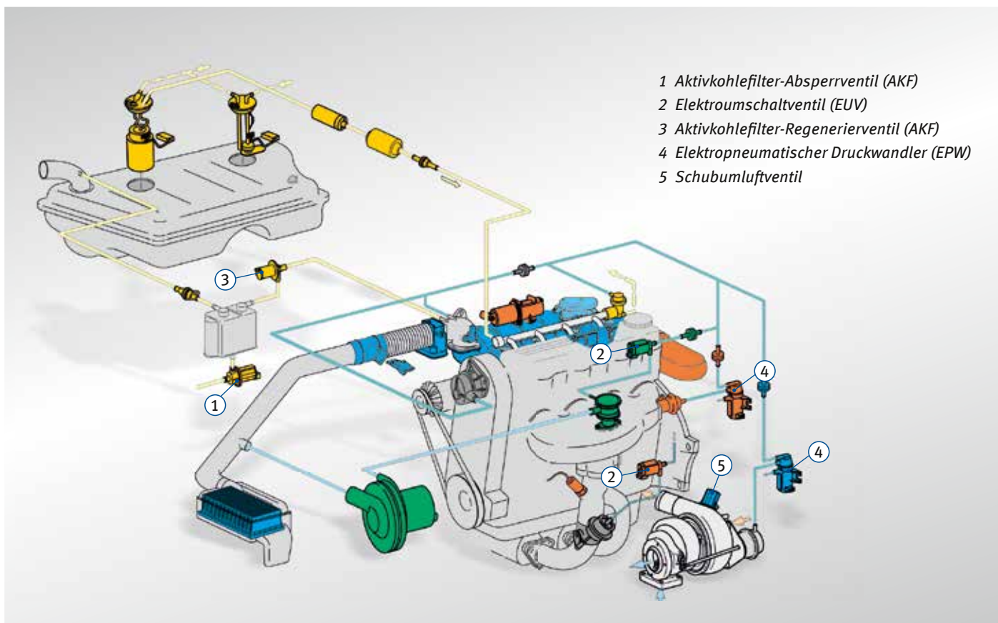
Abb. 1: Der Turbolader im motorischen Umfeld
