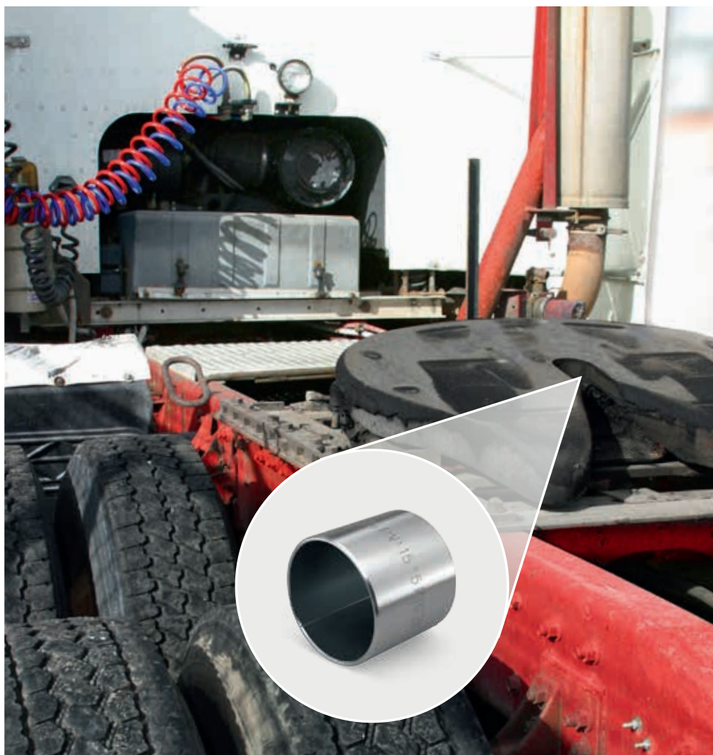
Supporto della ralla con boccole a strisciamento KS PERMAGLIDE® P10
