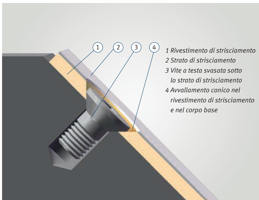
Fissaggio mediante foratura e avvitamento
