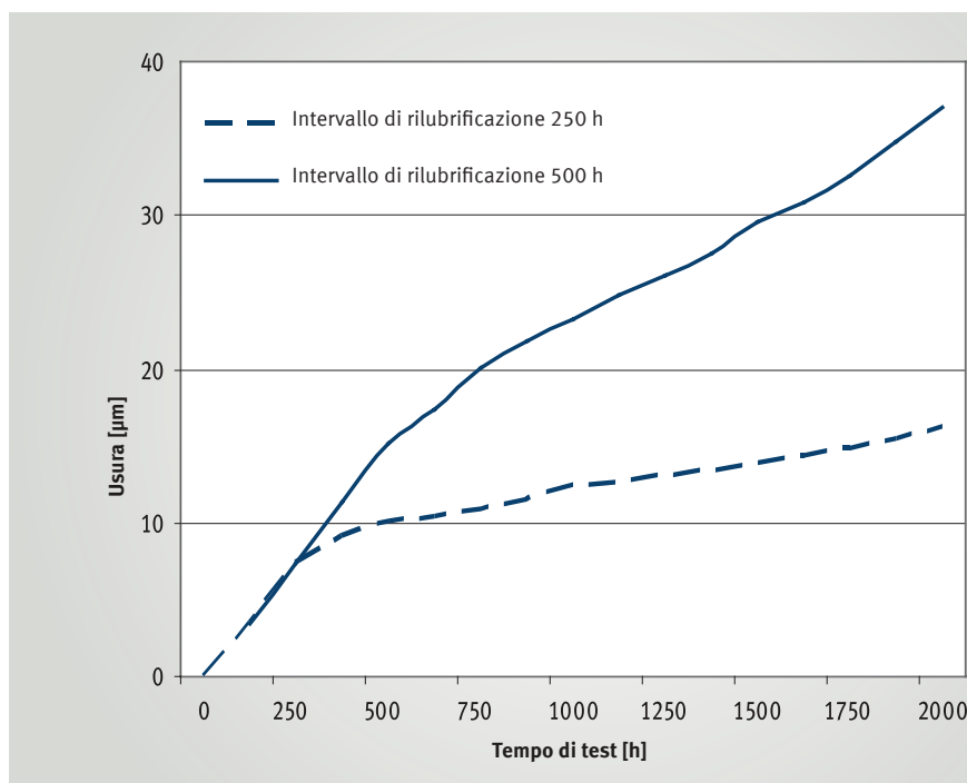
Curva dell'usura di un cuscinetto a strisciamento P2 (rappresentazione schematica)
