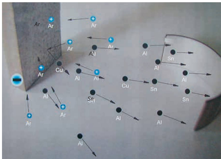
Fig. 2 proceso Sputter
