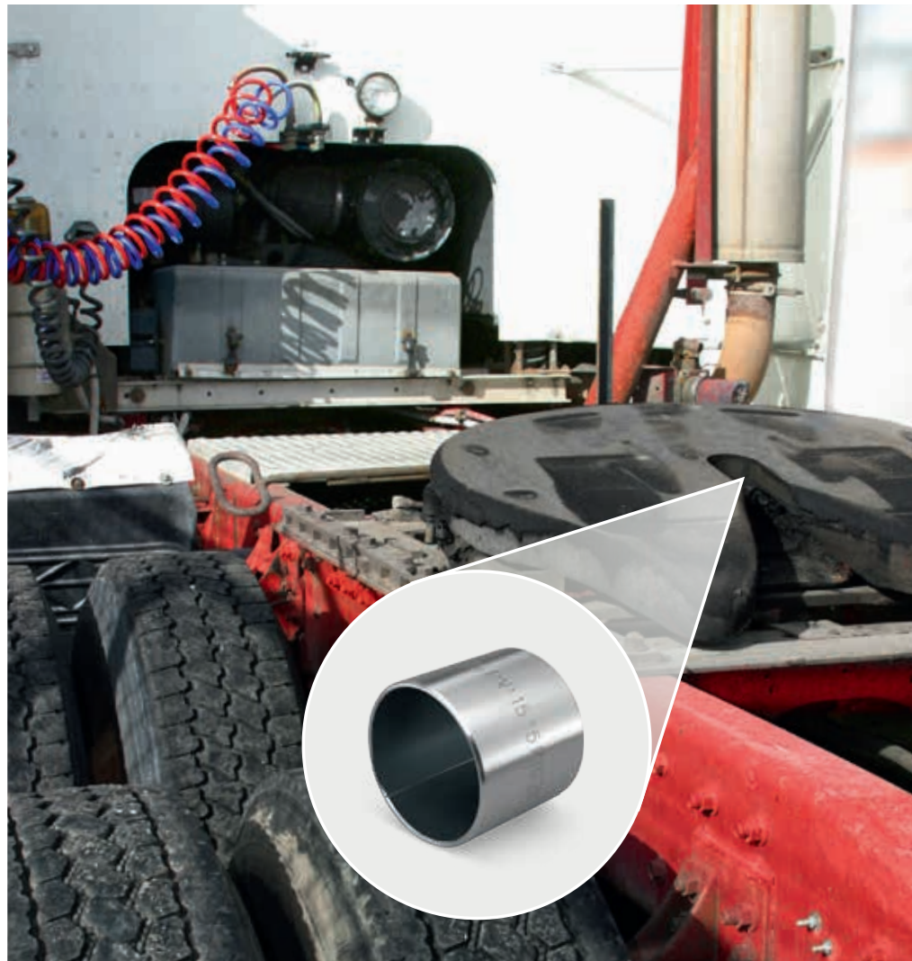
Palier de sellette d'attelage avec des bagues de coussinet KS PERMAGLIDE® P1
