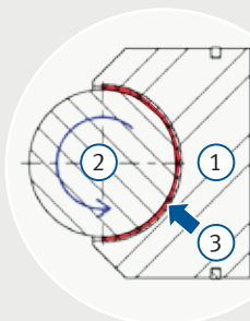
Application du principe de piston radial
