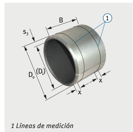
Fig. 2: Líneas de medición para la comprobación del espesor de la pared (ejemplo)
