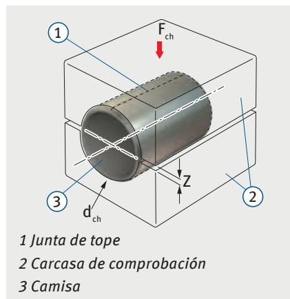
Fig. 1: Comprobación del diámetro exterior de la camisa D_o
