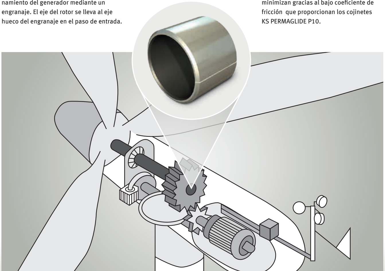
Los cojinetes KS PERMAGLIDE® P10 se emplean como cojinetes guía del eje del rotor en el engranaje de los sistemas eólicos
