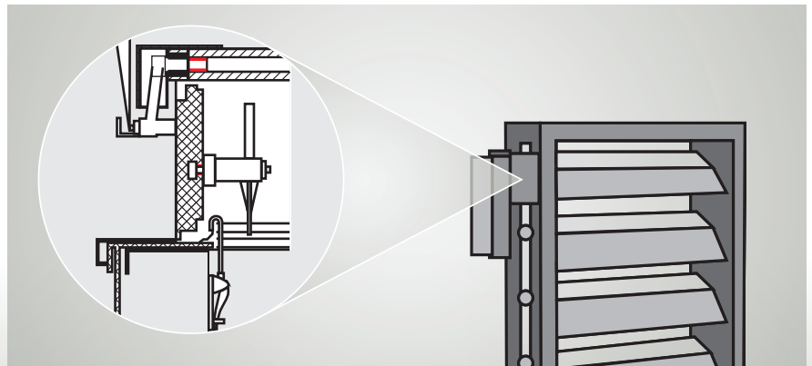
Alojamiento de las láminas mediante cojinetes KS PERMAGLIDE® P10
