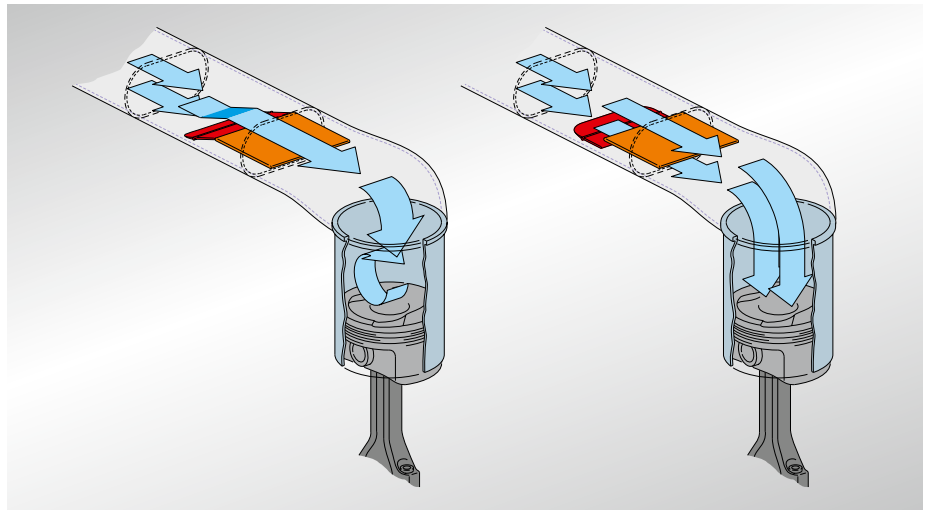
Clapet tumble : tourbillon vertical par rapport au sens de l'axe du piston à gauche : mode charge stratifiée ; à droite : mode homogène
