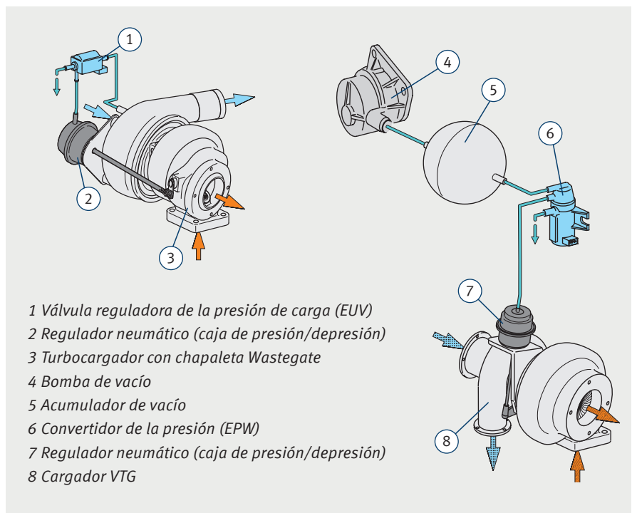
Ejemplo: cargador VTG y EPW (resaltado a color rojo) en el Audi A4 TDI
