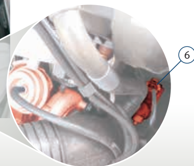
Ejemplo: cargador VTG y EPW (resaltado a color rojo) en el Audi A4 TDI
