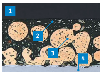
Composition de la surface de glissement à l'état initial
