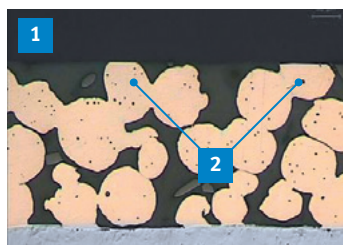
Composition de la surface de glissement à la fin du rodage
