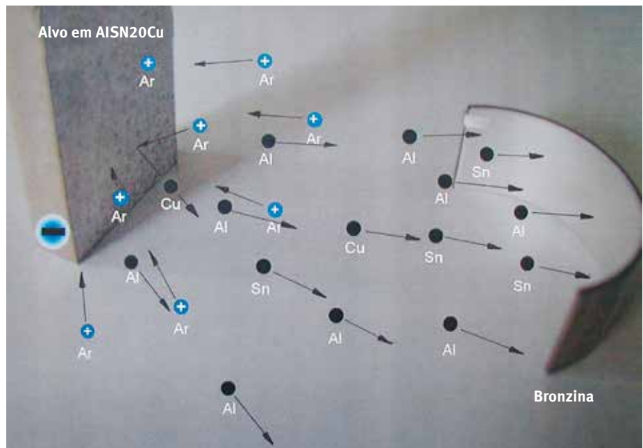
Fig. 2 Processo sputter
