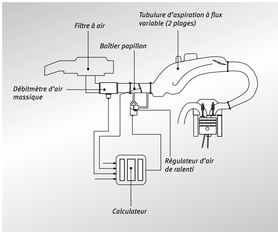
Fig. 39 Alimentation en air (schématique)
