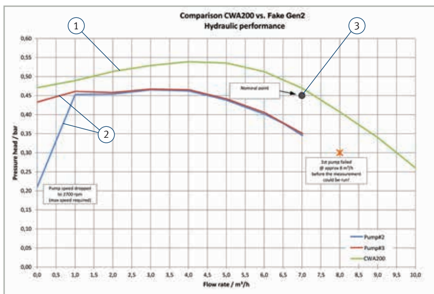
Medición hidráulica comparativa en el laboratorio de pruebas de PIERBURG (documento original) – (1) PIERBURG CWA 200, (2) falsificaciones, (3) punto de diseño del fabricante de vehículos
