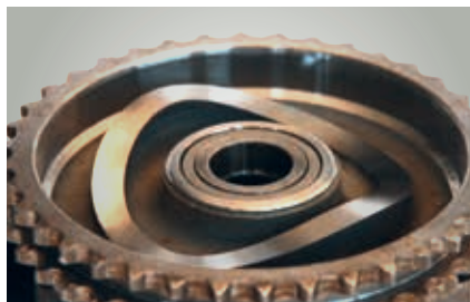
Исправный эксцентрик
