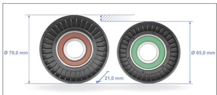
Bild 2: Umlenkrolle 532 0404 30 für Fahrzeuge mit Ottomotor (links) und Umlenkrolle 532 0406 30 für Fahrzeuge mit Dieselmotor (rechts)
