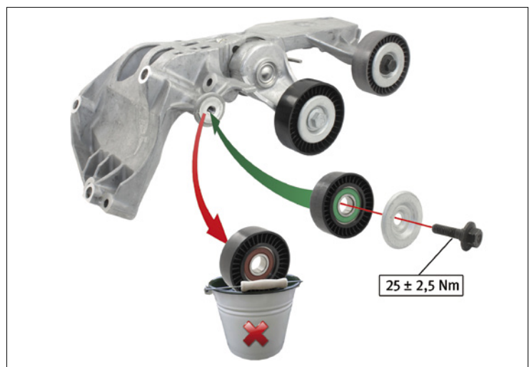
Bild 1: Spanneinheit 534 0243 10
