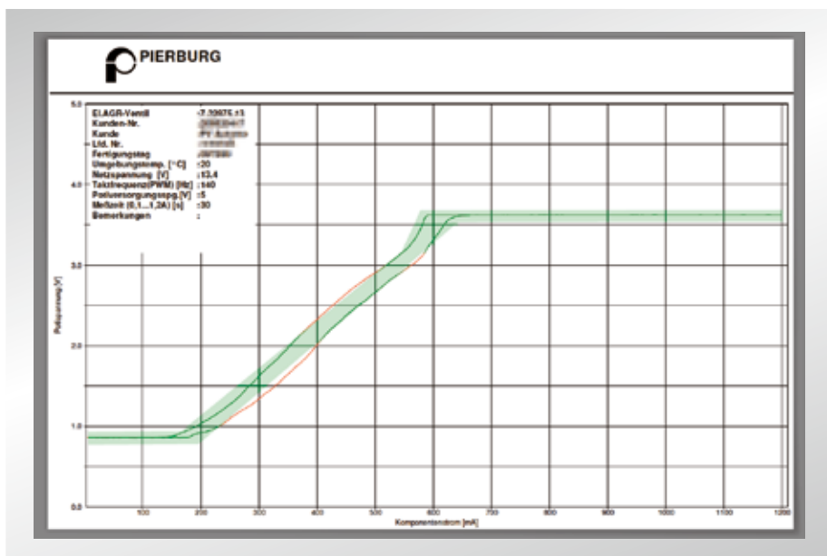
Fig. 1: Folha de dados original; intervalo de regulação (a título de exemplo) destacado a verde
