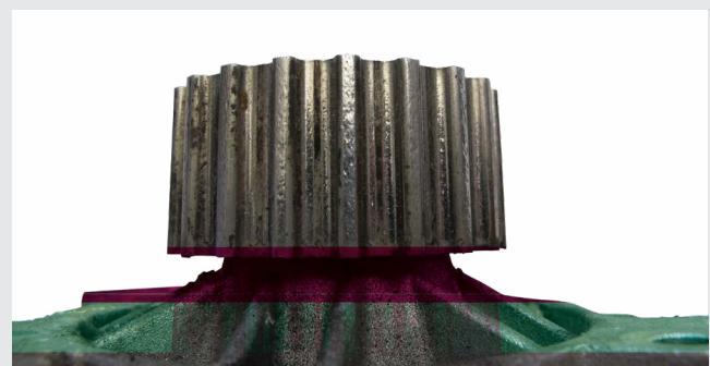
Uszkodzone przez zabrudzenia i zużycie koło napędowe (uszkodzenia łożyska)
