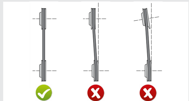
Błędy zbieżności paska
