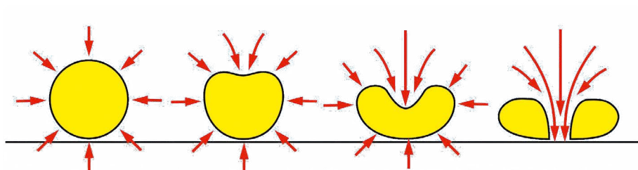
Powstawanie pęcherzyków i ich rozpad
