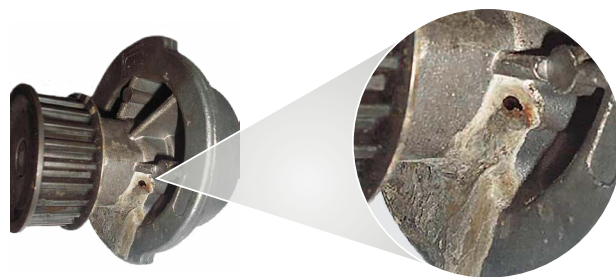
Pompa wodna nieszczelna wskutek wody zawierającej kamień
