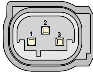
4.07360.53.0 adaptör kablosunun konnektör görünümü
