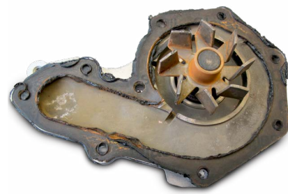
Utilização excessiva de produtos de vedação líquidos (neste caso, silicone)
