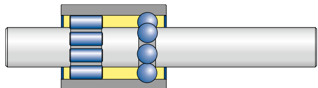
Fig. 2: Rolamento de esferas e rolos
