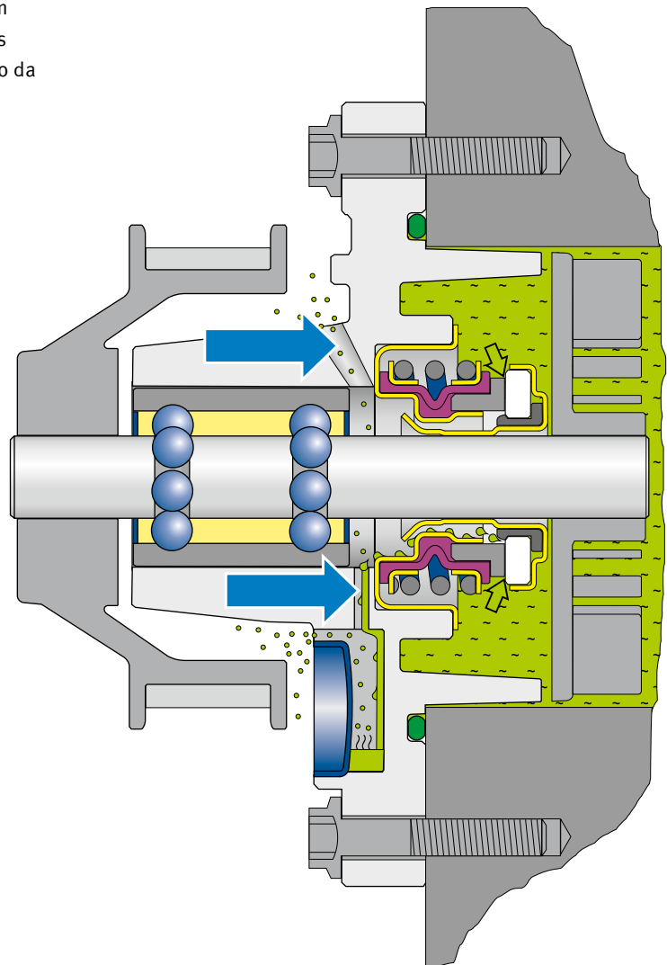
Orifício de ventilação e de vazamento
