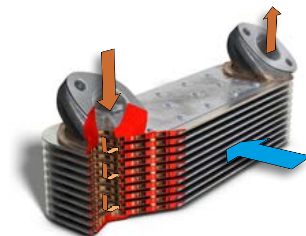
Radiatore dell'olio per veicoli commerciali
