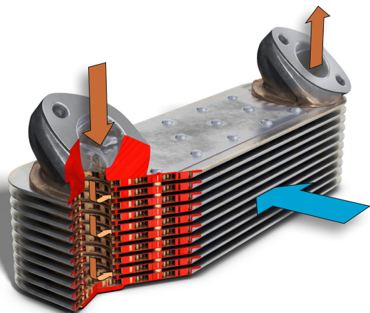
Nkw-Ölkühler
