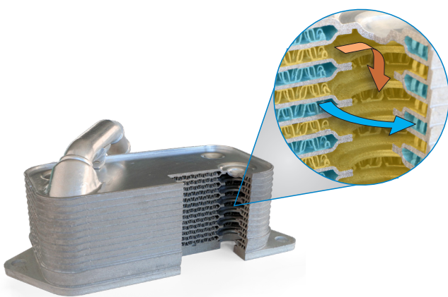
Pkw-Ölkühler
