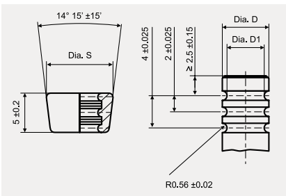
Mehrrillenkegelstück MK 5-6, Konus 1:4
