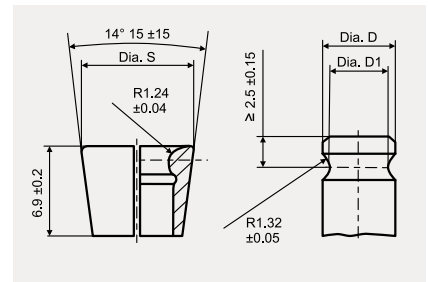
أجزاء مخروط الحزوز LK، مخروط ١:٤
